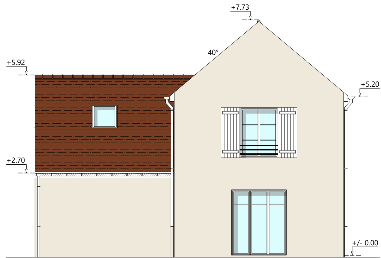
Façade Sud
