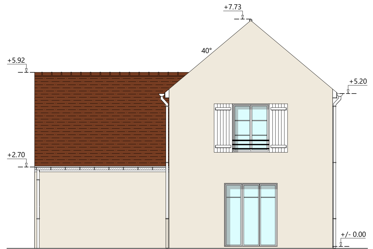
Façade Sud
