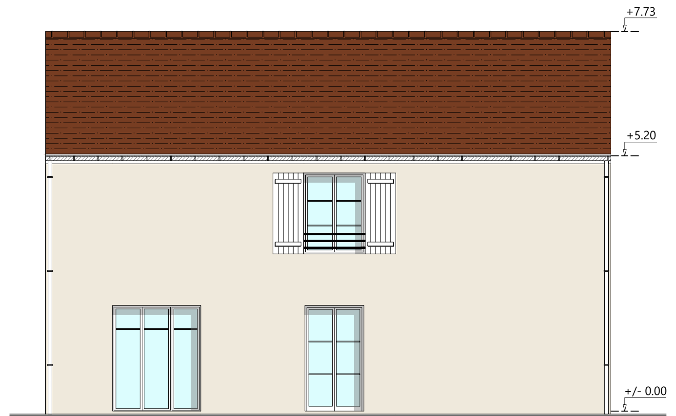
Façade Est
