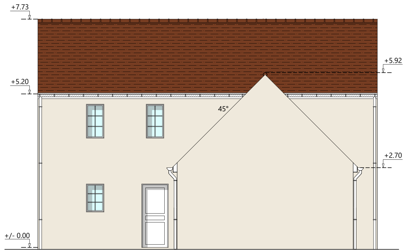
Façade Ouest
