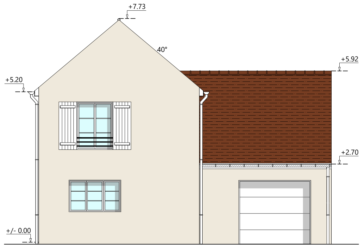
Façade Nord
