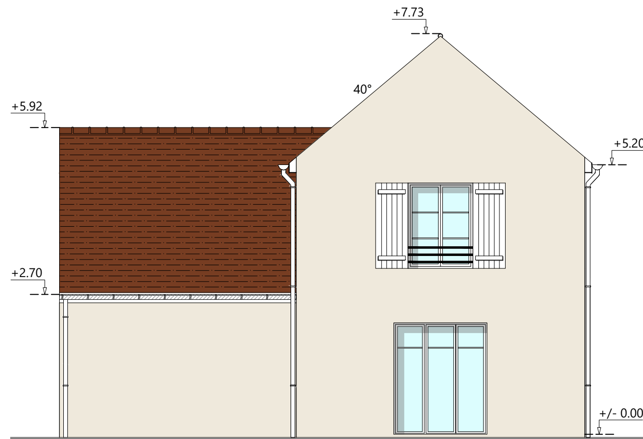
Façade Sud
